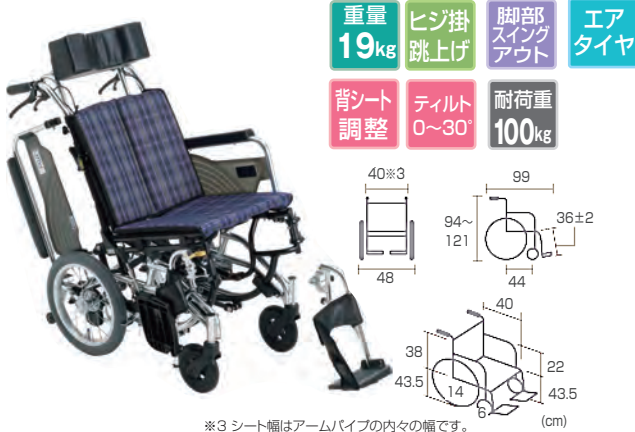
※3 シート幅はアームパイプの内々の幅です。
